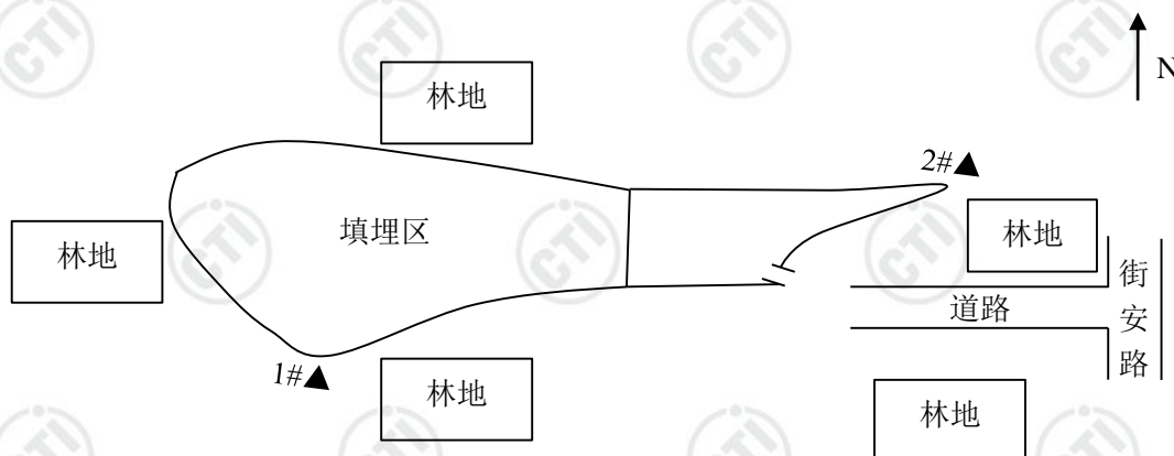
附: 厂界噪声测点示意图
